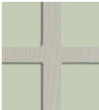
DETALLE CRISTALERA SERIE FRANCESA SIN JUNQUILLO PMJJ
